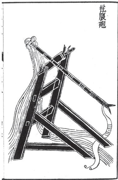
图七 北宋拄腹砲和合砲
